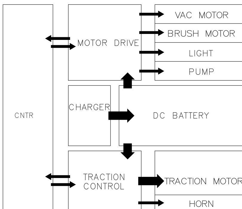
Schaltbild
